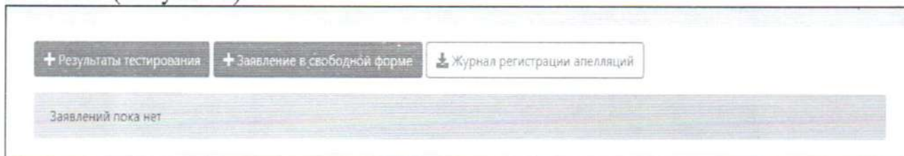
Рисунок 2 - Интерфейс Системы
